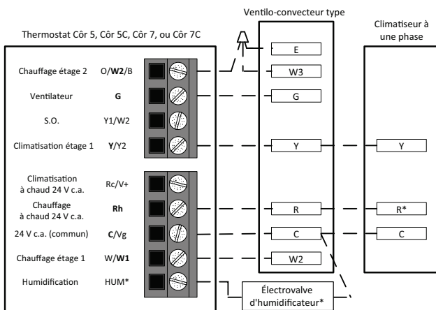
Fig. 12 – Ventilo-convecteur type avec climatiseur
