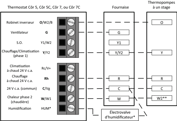
Fig. 18 – Chaudière à une phase avec thermopompe (chauffage hybride)
