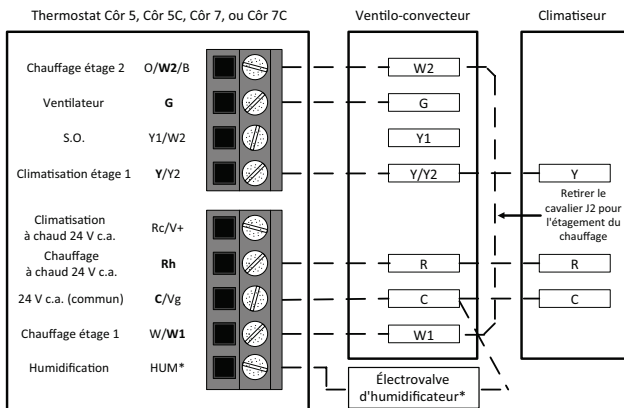
Fig. 15 – Ventilo-convecteur FV et FK avec climatiseur à 1 phase
