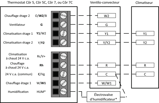
Fig. 11 – Ventilo-convecteur FV et FK avec climatiseur à 2 phases
