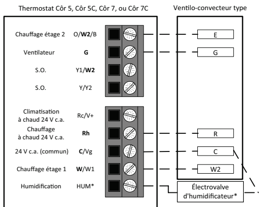
Fig. 14 – Chauffage par ventilo-convecteur type seulement
