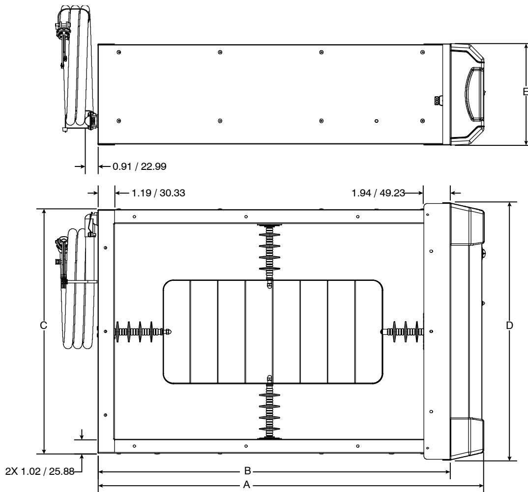
Fig. 21 - Dimensions
