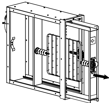
Fig. 7 - Removing FEM
