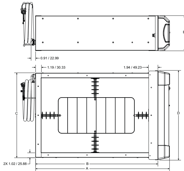
Fig. 21 - Dimensions
