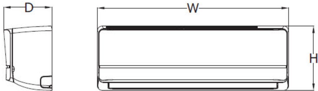
Fig. 2 – Indoor Unit
