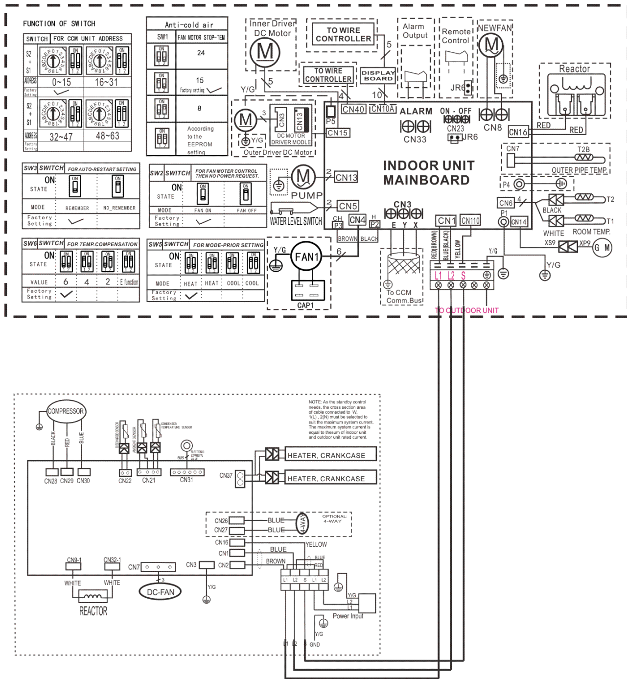
Fig. 6 – Wiring Diagram 38MAQB09---3 / 40MBQ09C---3 AND 38MAQB12---3 / 40MBQ12C---3
