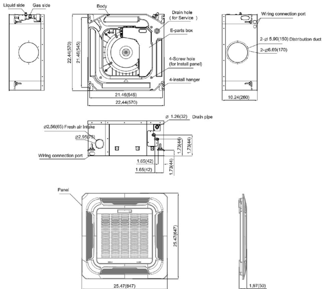
Fig. 1 – Indoor unit
