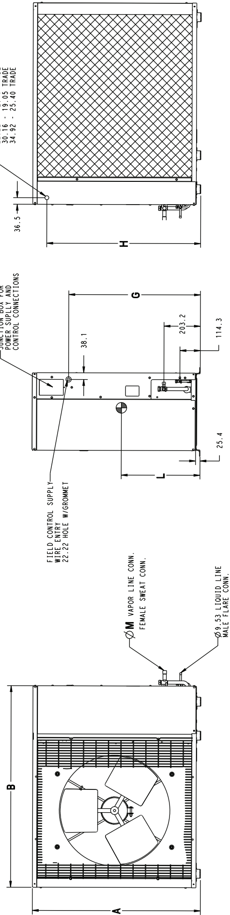
Fig. 8 - 38QRR Dimensions - SI
