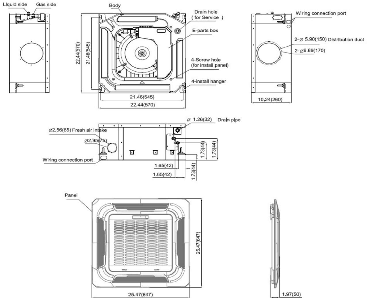
Fig. 1 – Indoor unit
