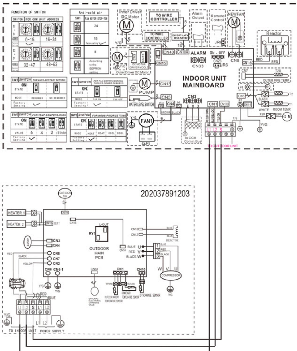
Fig. 7 – Wiring Diagram 38MAQB18---3 / 40MBQ18C--3
