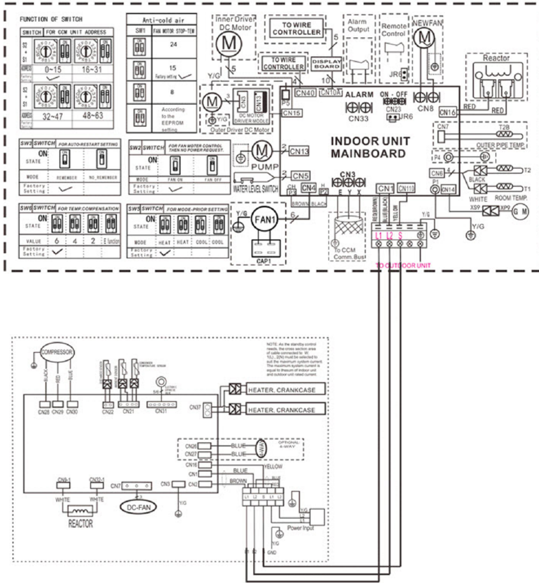
Fig. 6 – Wiring Diagram 38MAQB09---3 / 40MBQ09C---3 AND 38MAQB12---3 / 40MBQ12C---3
