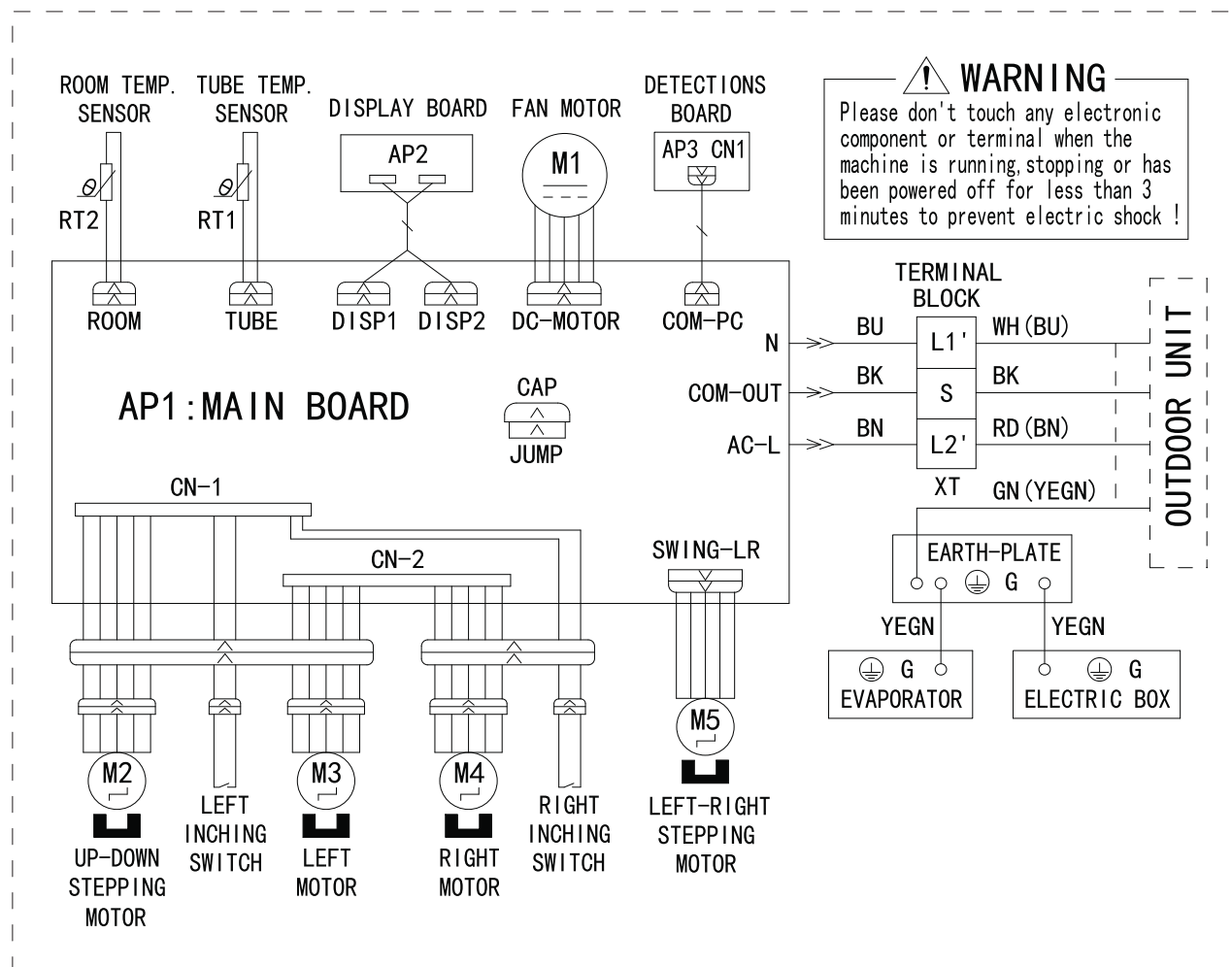
Fig. 13 – Indoor unit
