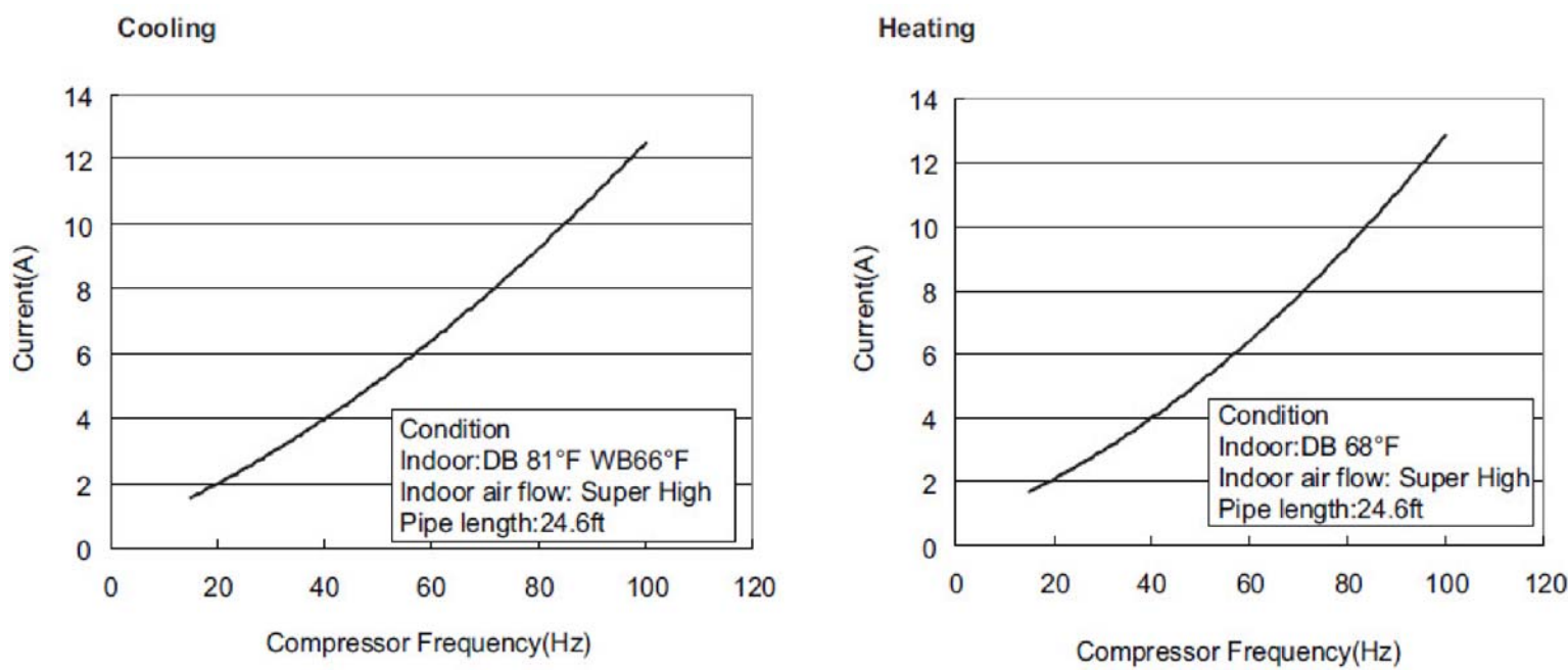
Fig. 8 - 18K
