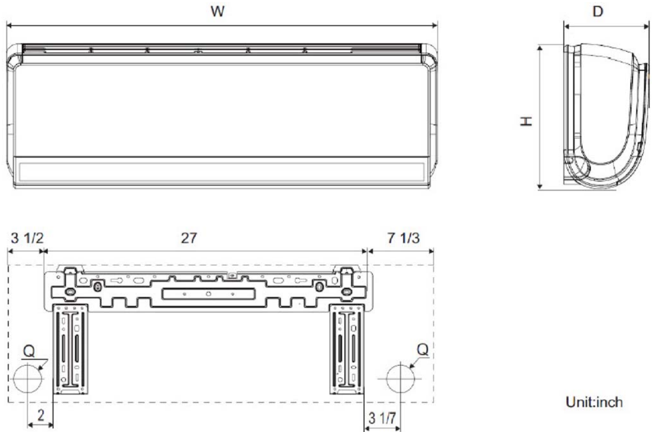
Fig. 2 – Indoor unit
