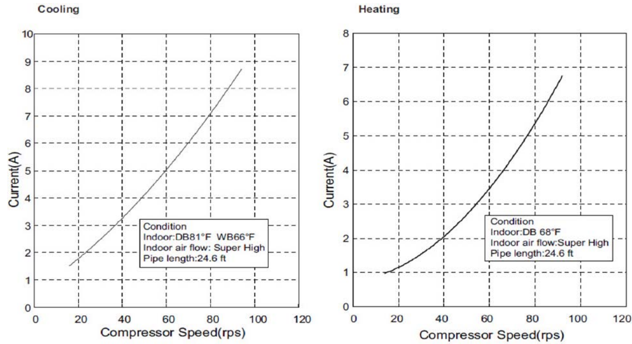
Fig. 7 - 09K/12K
