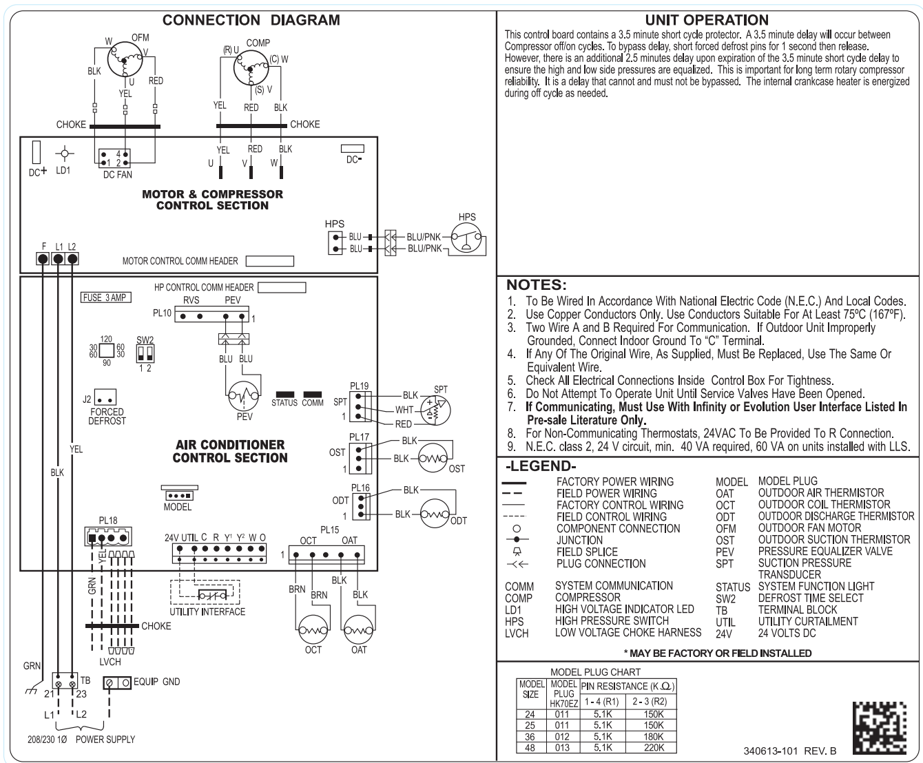
Fig. 1 – 24VNA9 208/230-1
