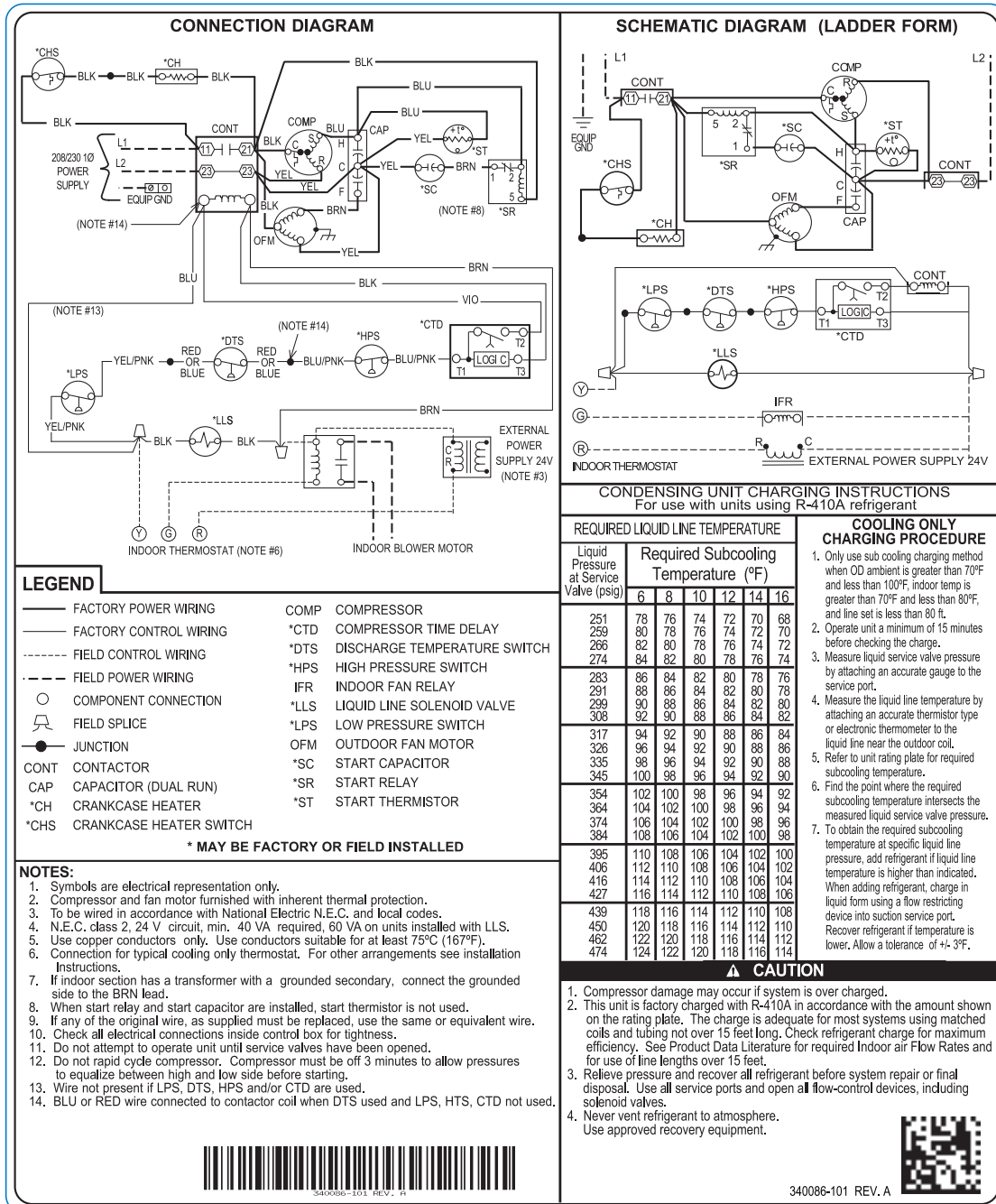
Fig. 1 – Wiring Diagram — Models BA16N*018-030 / BA13NA, BA14NA, BA15NA018-060, 208/230-1
